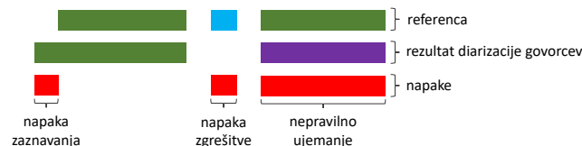
Slika 2: Pri vrednotenju diarizacije upoštevamo tri različne vrste napak. Njihov časovni delež v delih posnetka, v katerih je prisoten govor, je mera DER.
